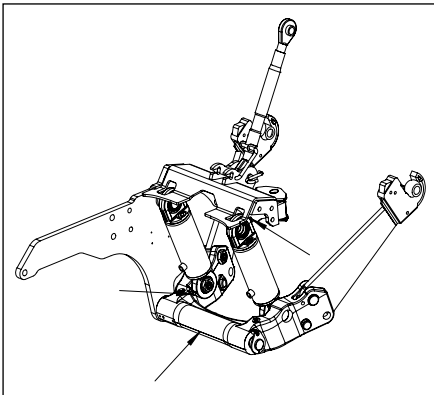
Slika 7.1 Mazalne točke
