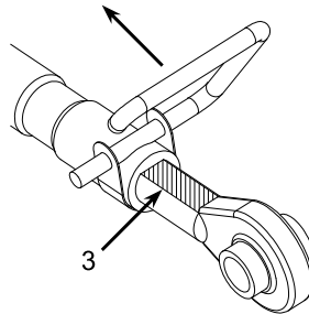
Fig. 6.8: Låsebøjle
