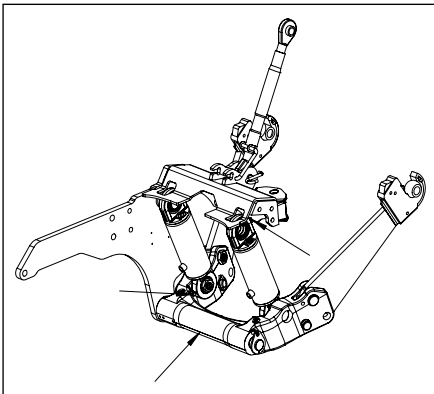
Bild 7.1: Fettpunkter
