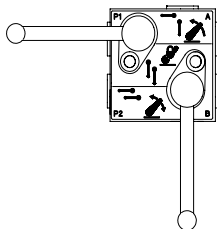
Sl. 6.1: Pojedinačni rad prednjeg podizača.
