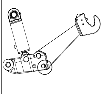
Fig. 6.4: flydestilling
