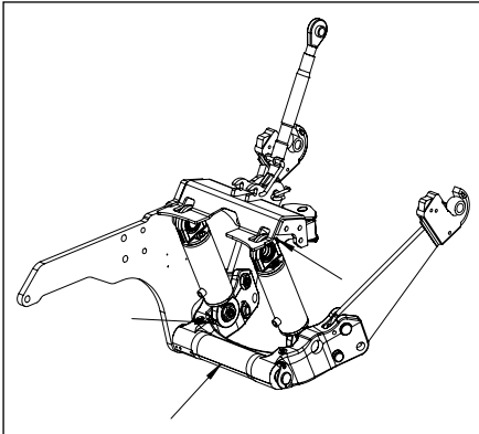
Fig 7.1: smøreplerner (smøre punkter)
