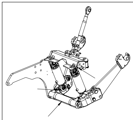
Ilustración 7.1: Puntos de engrase
