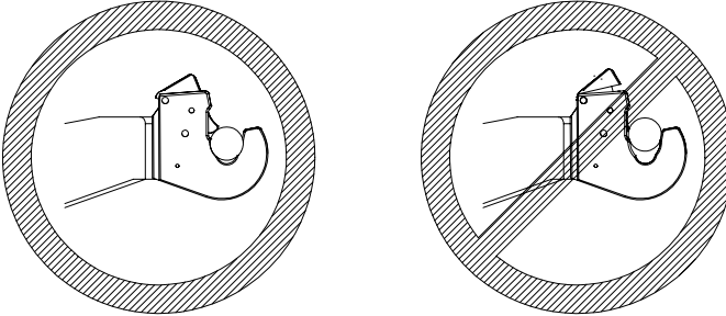
Kuva 6.9: Kuulien lukitus
