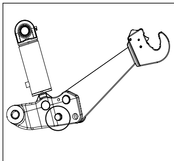
Fig. 6.5: Posição fixa
