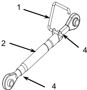
Obr. 6.7: horní kloub
