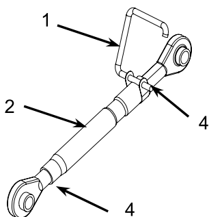
Bild 6.7: Övre stag
