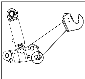
Fig. 6.4: Posição oscilante
