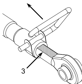
Rys. 6.8: blokada trzpienia obrotowego
